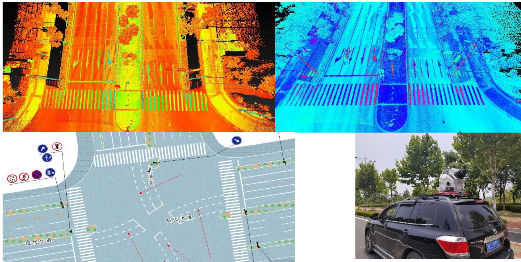
徕卡Pegasus:Two
